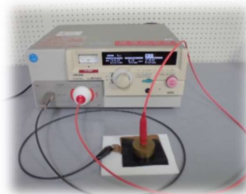
たいでんあつしけんき 耐電圧試験器
